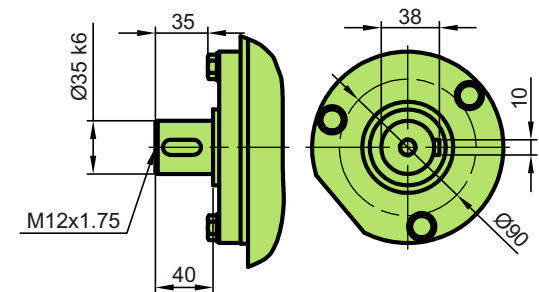
Eje / Shaft B
