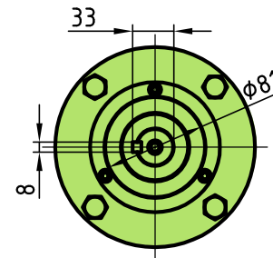
Eje opcional / Optional shaft B
